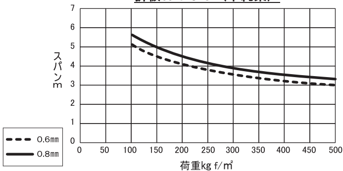
折板W150 (片持梁)
