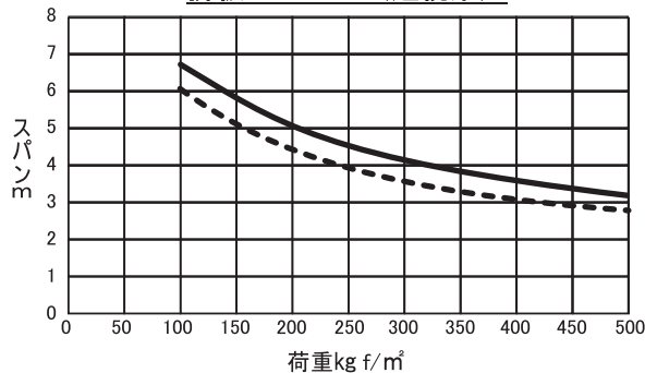
折板W150 (連続梁)
